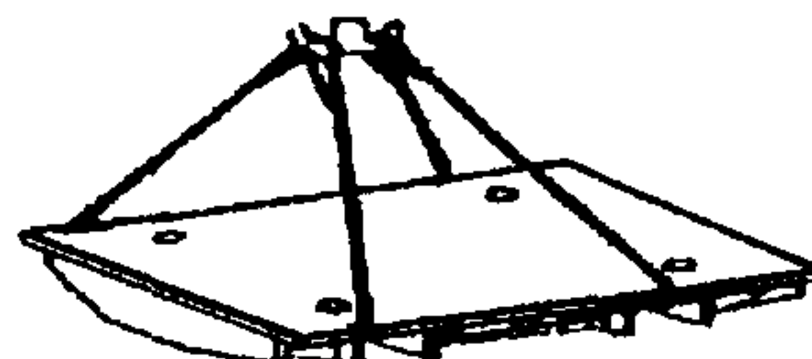
Схема строповки рамы тележки
