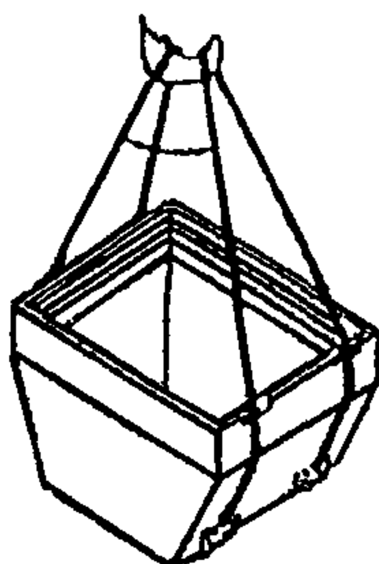
Схема строповки короба
