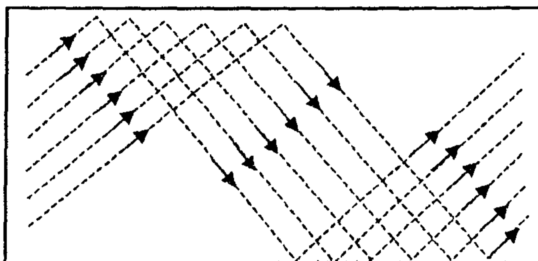
Рис. 13. Зигзагообразные швы
