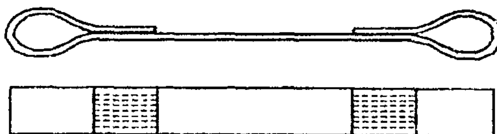
Рис. 1. Одиночный петлевой строп с мягкими плоскими петлями
