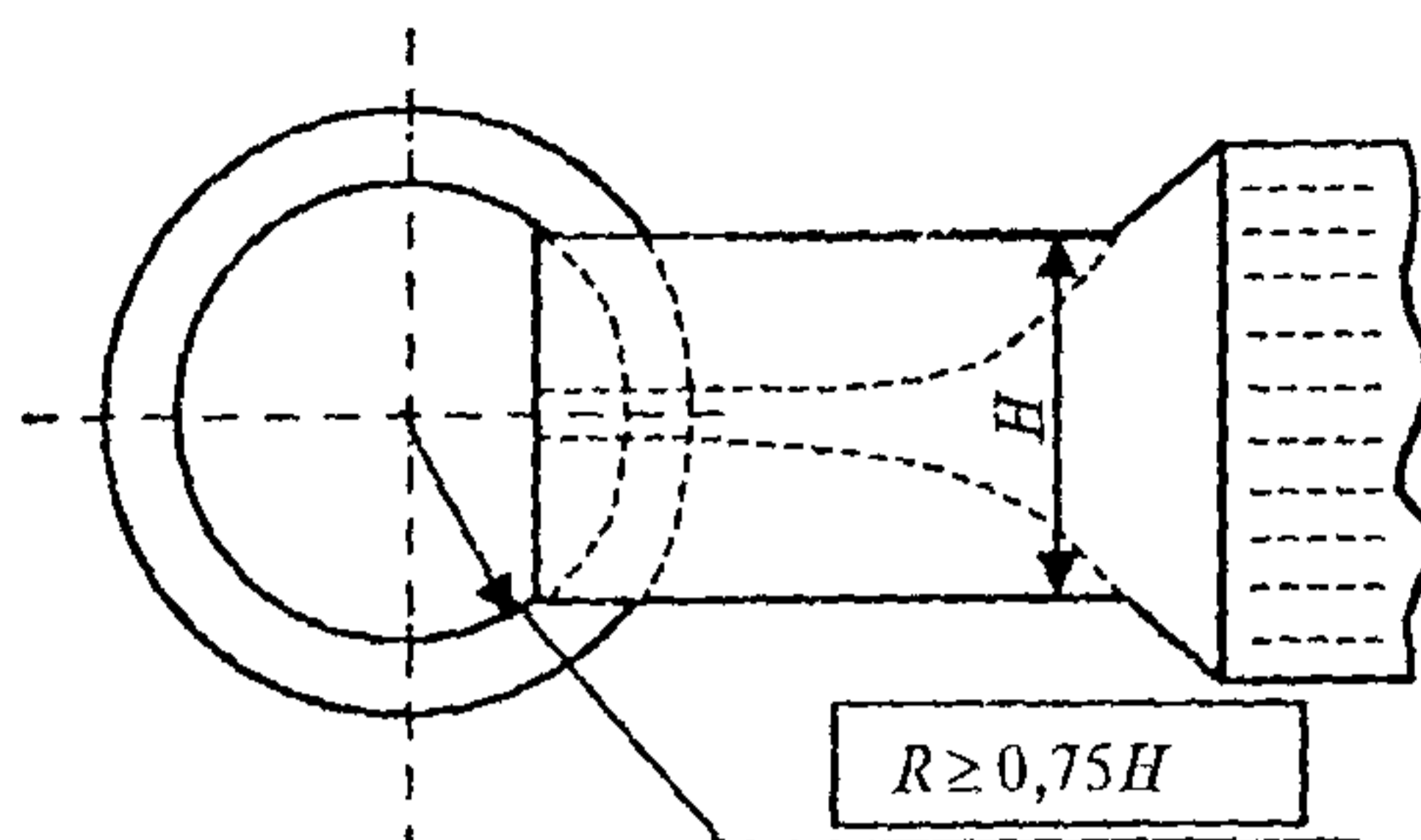
Рис. 16. Назначение радиуса кривизны для стропов из лент с H \leq 75 мм.
